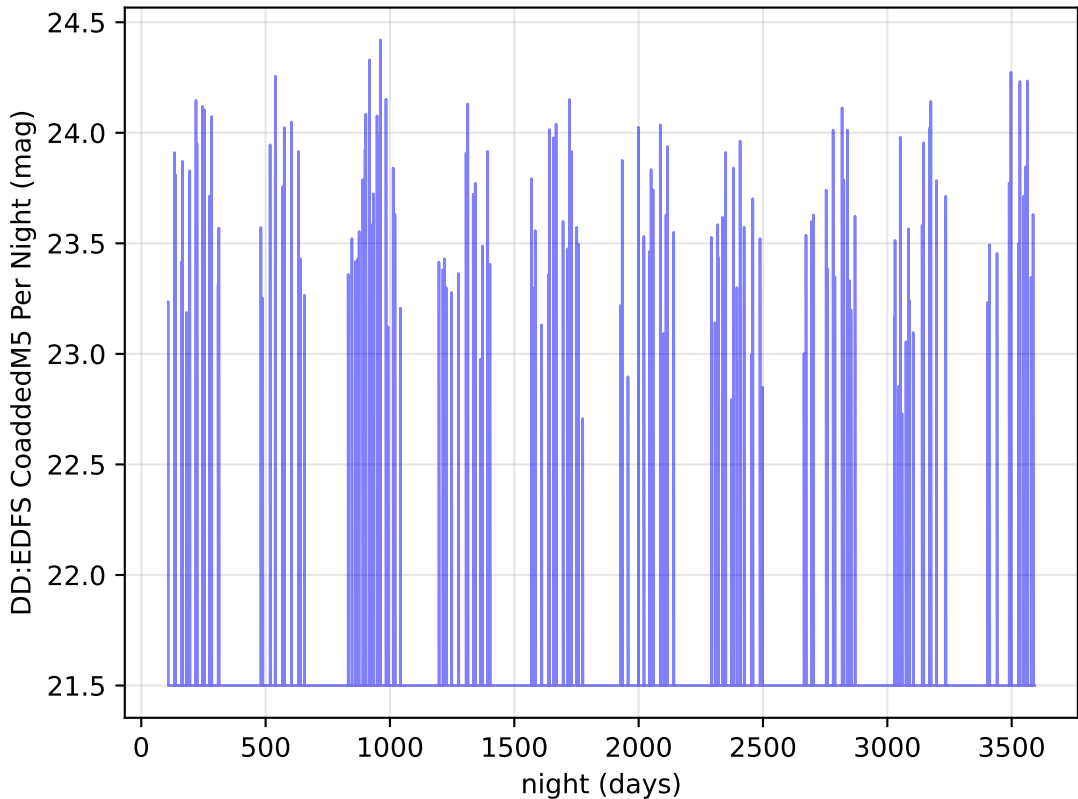
weather_cloudso30v3.5_10yrs y band: DD:EDFS CoaddedM5 Per Night
