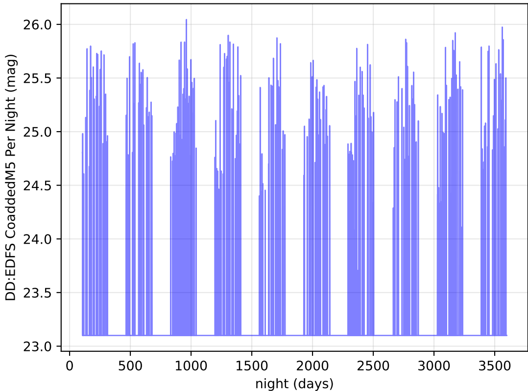
weather_cloudso30v3.5_10yrs i band: DD:EDFS CoaddedM5 Per Night
