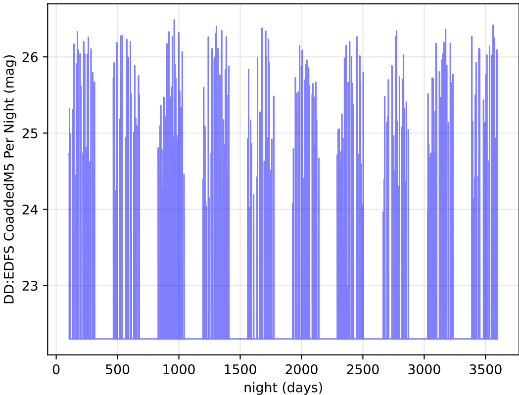
weather_cloudso30v3.5_10yrs g band: DD:EDFS CoaddedM5 Per Night
