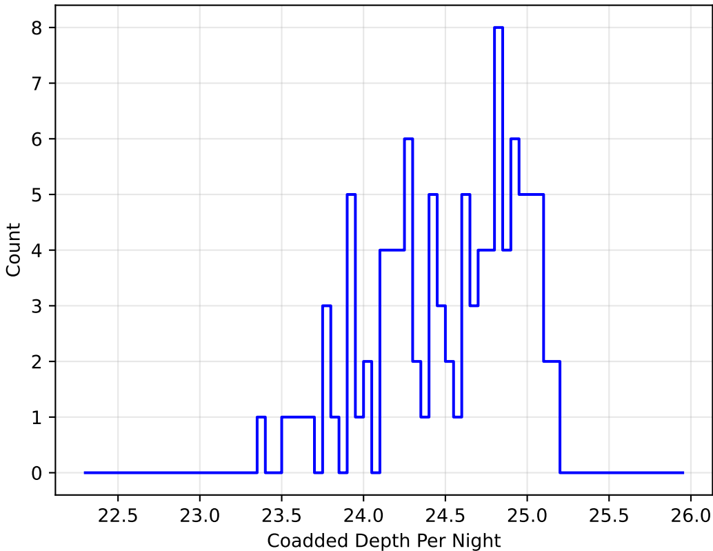
weather_cloudso30v3.5_10yrs u band: DD:EDFS CoaddM5PerNight
