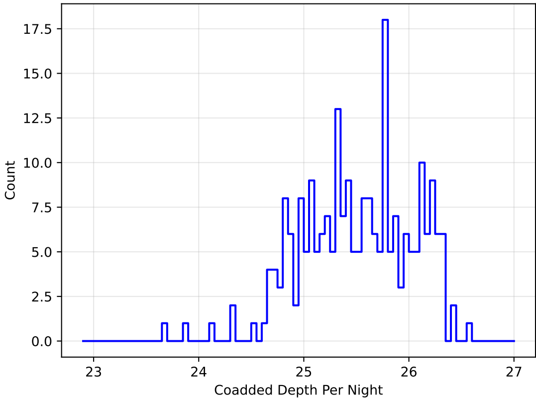
weather_cloudso30v3.5_10yrs r band: DD:EDFS CoaddM5PerNight
