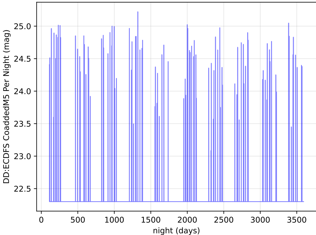
weather_cloudso30v3.5_10yrs u band: DD:ECDFS CoaddedM5 Per Night
