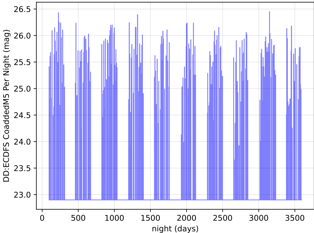
weather_cloudso30v3.5_10yrs r band: DD:ECDFS CoaddedM5 Per Night
