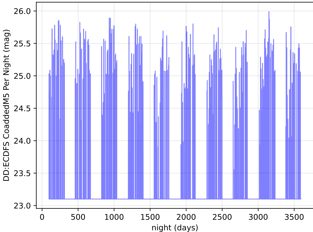
weather_cloudso30v3.5_10yrs i band: DD:ECDFS CoaddedM5 Per Night
