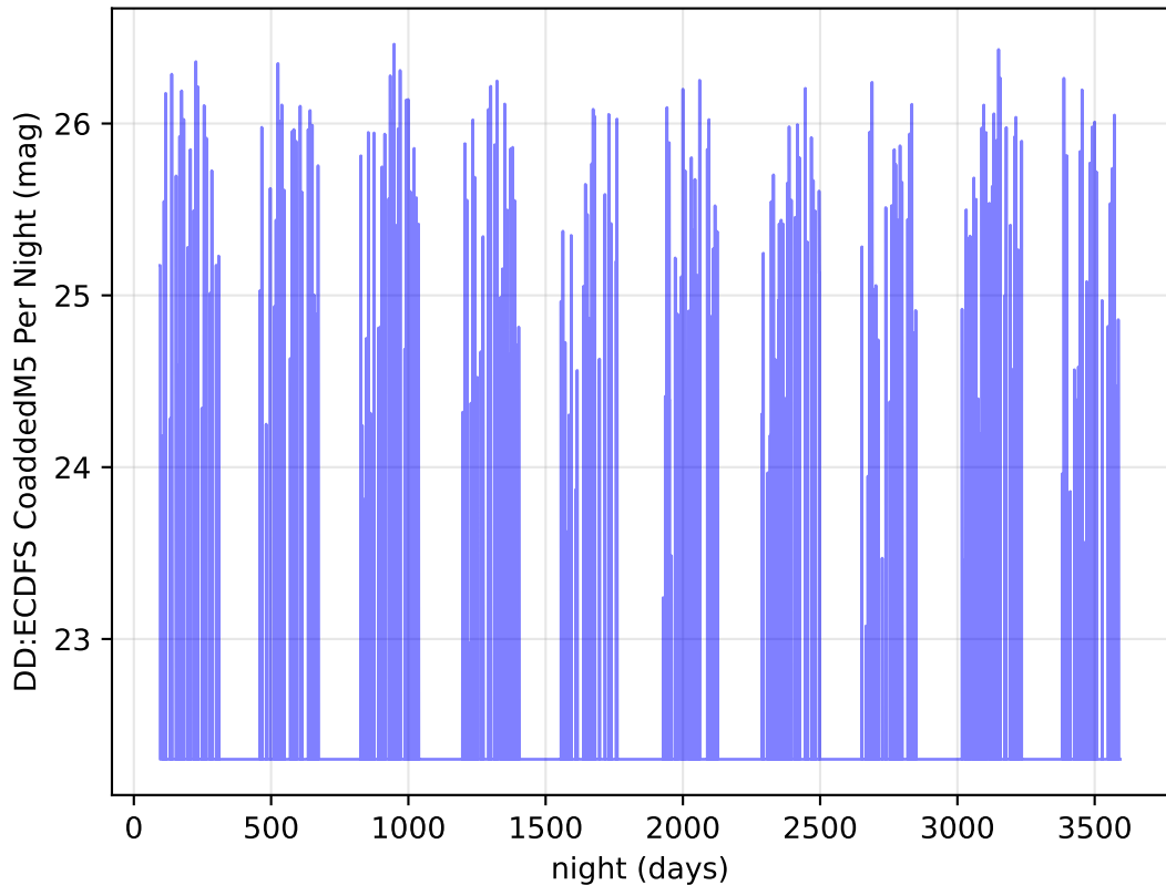
weather_cloudso30v3.5_10yrs g band: DD:ECDFS CoaddedM5 Per Night
