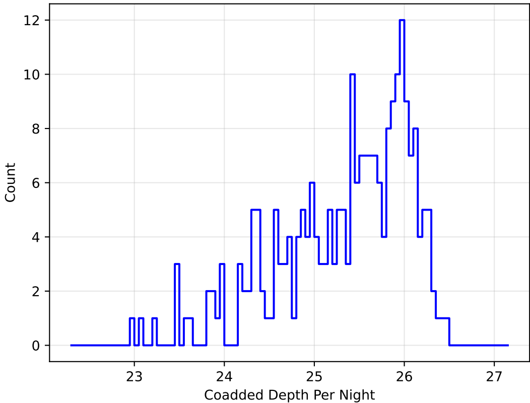
weather_cloudso30v3.5_10yrs g band: DD:ECDFS CoaddM5PerNight
