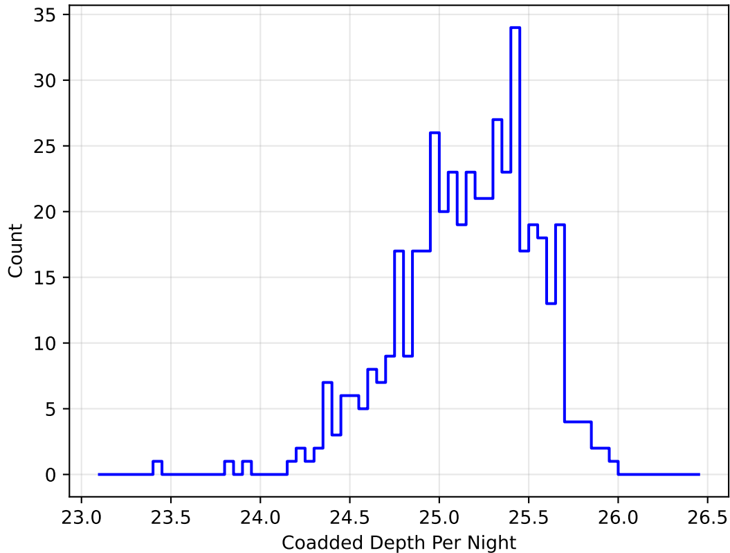
weather_cloudso30v3.5_10yrs i band: DD: COSMOS CoaddM5PerNight
