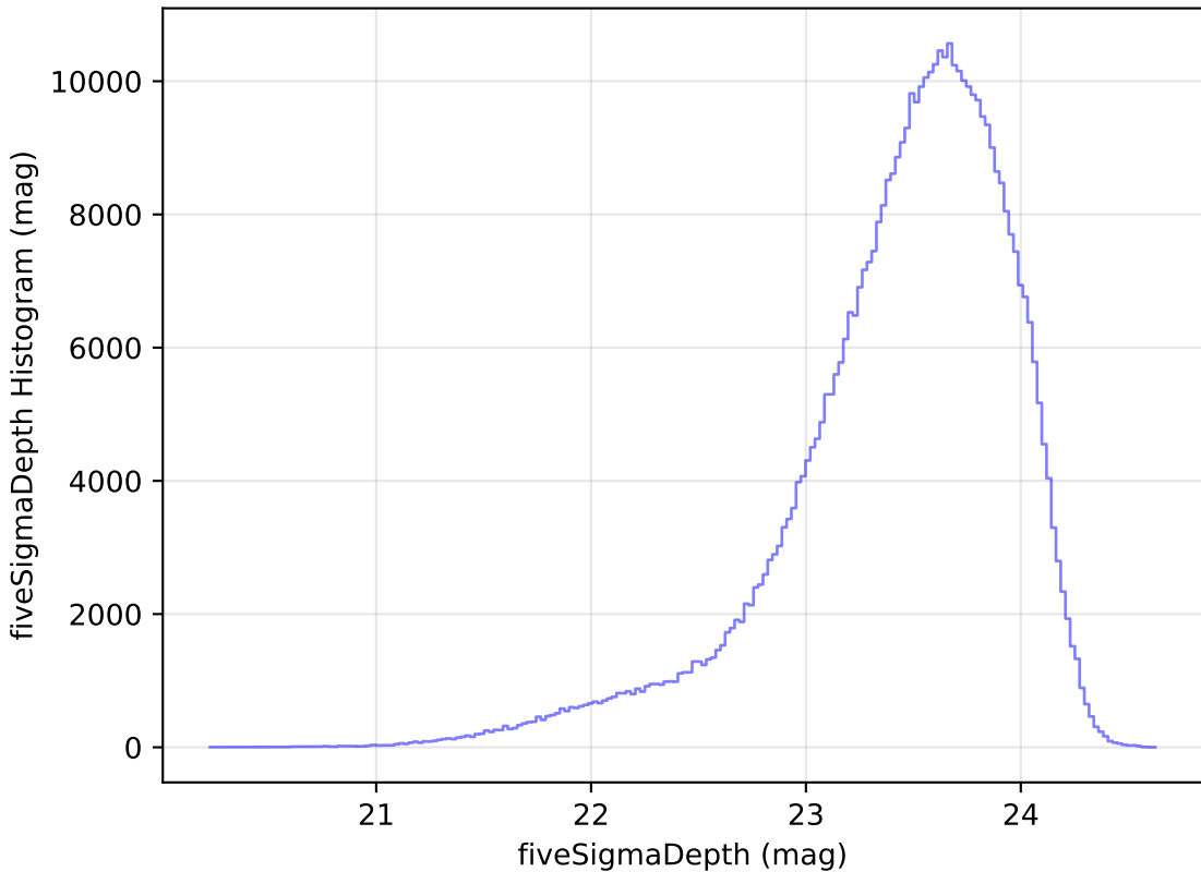
weather_cloudso30v3.4_10yrs i: fiveSigmaDepth Histogram
