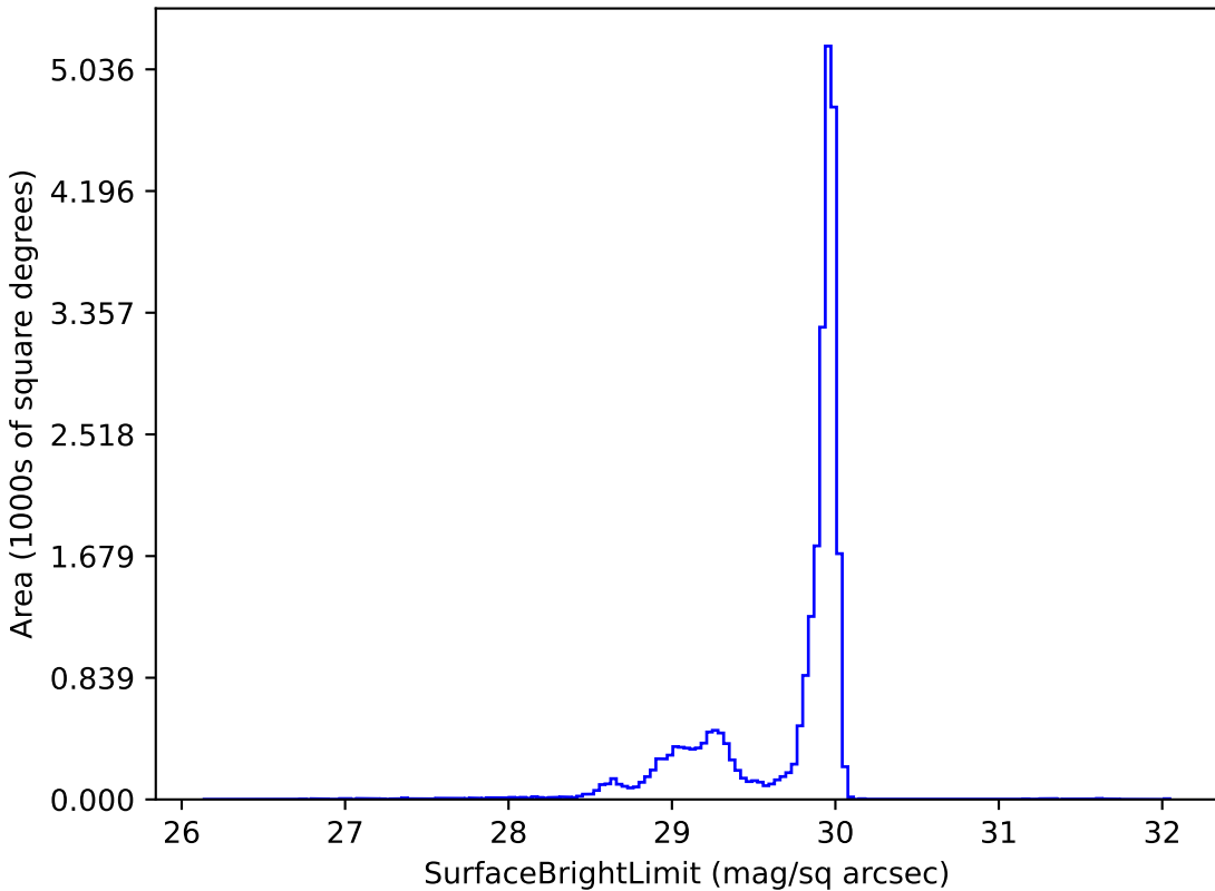
weather_cloudso30v3.4_10yrs i: SurfaceBrightLimit
