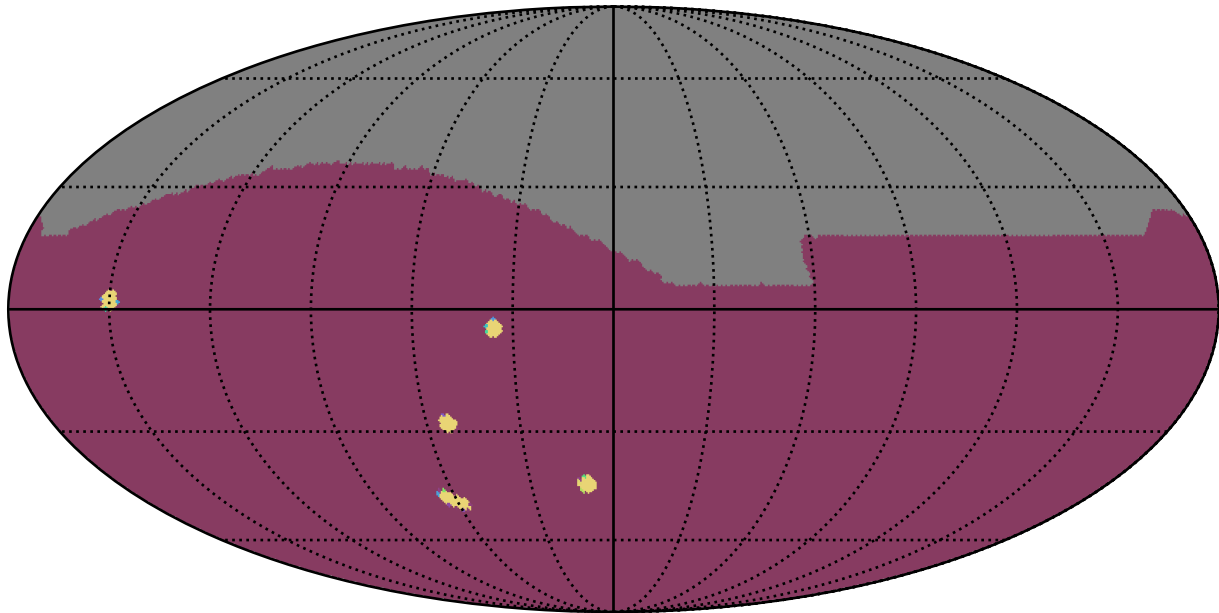
weather_cloudso30v3.4_10yrs : NumberOfQuickRevisits
