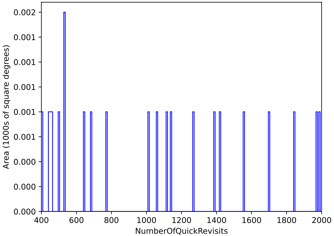
weather_cloudso30v3.4_10yrs : NumberOfQuickRevisits
