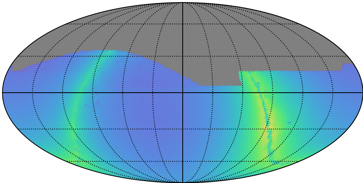
weather_cloudso30v3.4_10yrs z: Nstars_no_crowding
