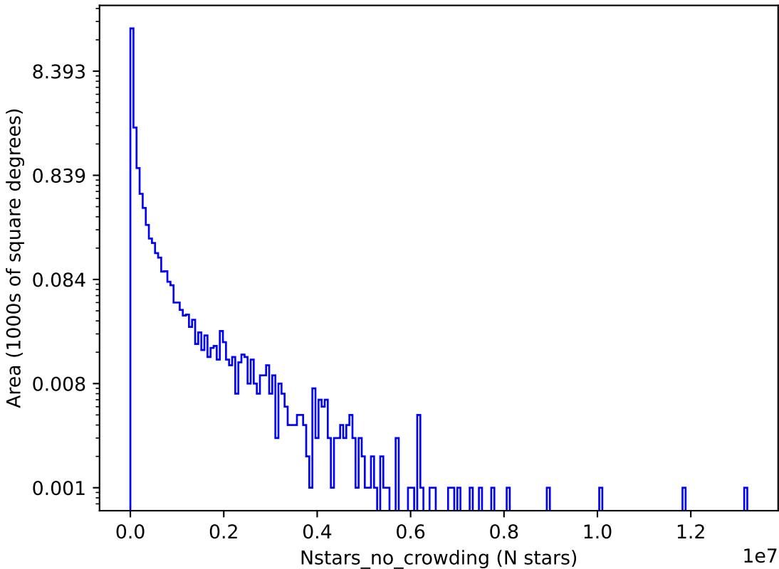
weather_cloudso30v3.4_10yrs g: Nstars_no_crowding
