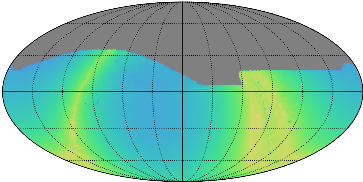
weather_cloudso30v3.4_10yrs i: N stars to Precision 0.20
