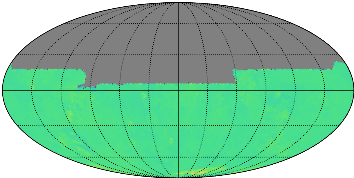
weather_cloudso30v3.4_10yrs y: Kuiper rotTelPos
