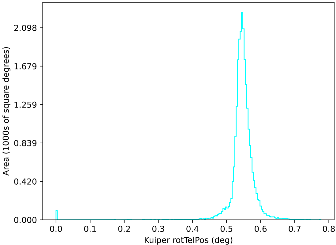
weather_cloudso30v3.4_10yrs u: Kuiper rotTelPos
