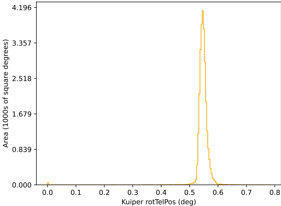
weather_cloudso30v3.4_10yrs r: Kuiper rotTelPos
