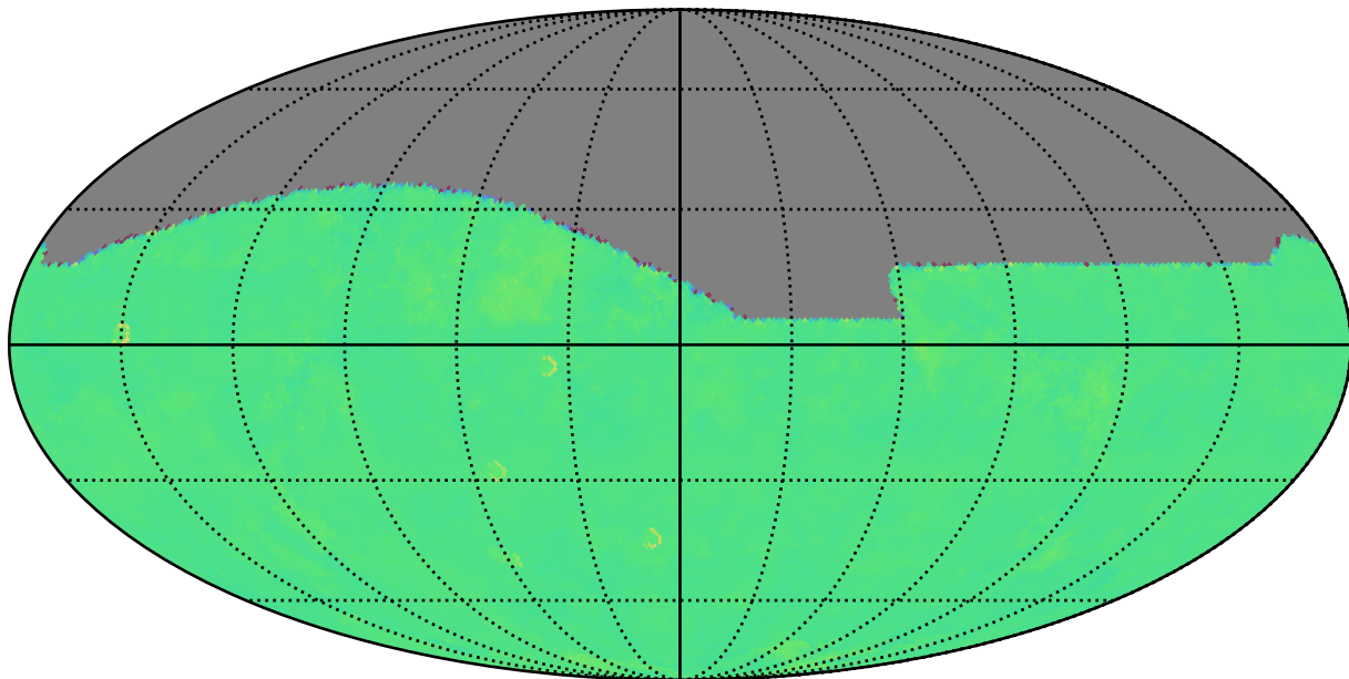
weather_cloudso30v3.4_10yrs i: Kuiper rotTelPos
