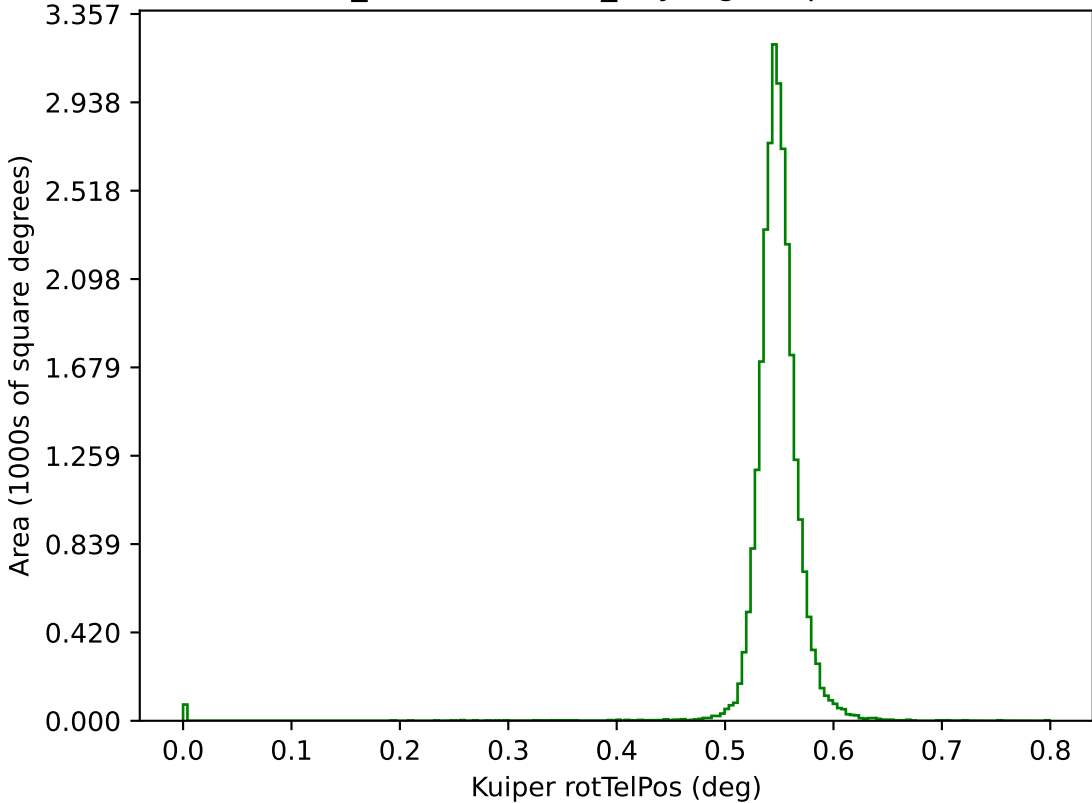
weather_cloudso30v3.4_10yrs g: Kuiper rotTelPos
