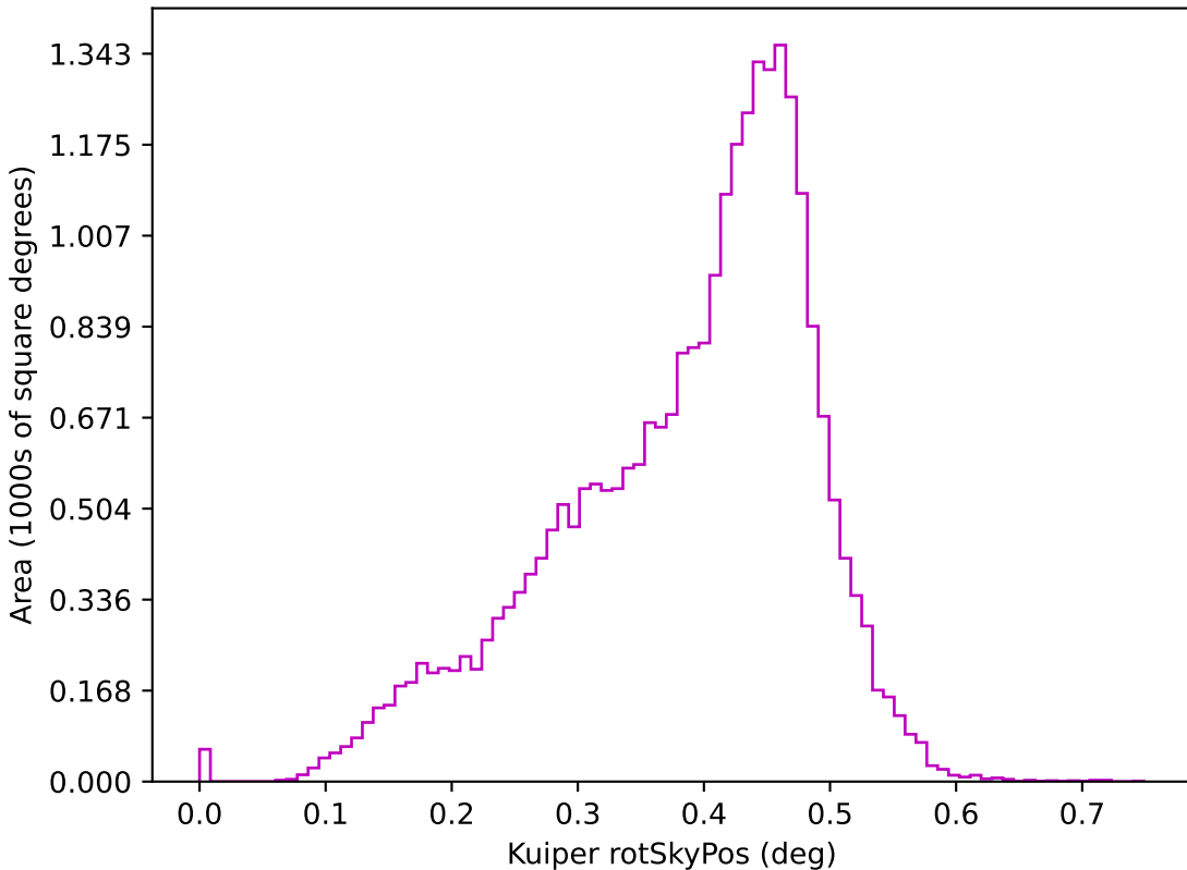
weather_cloudso3v3.4_10yrs z: Kuiper rotSkyPos
