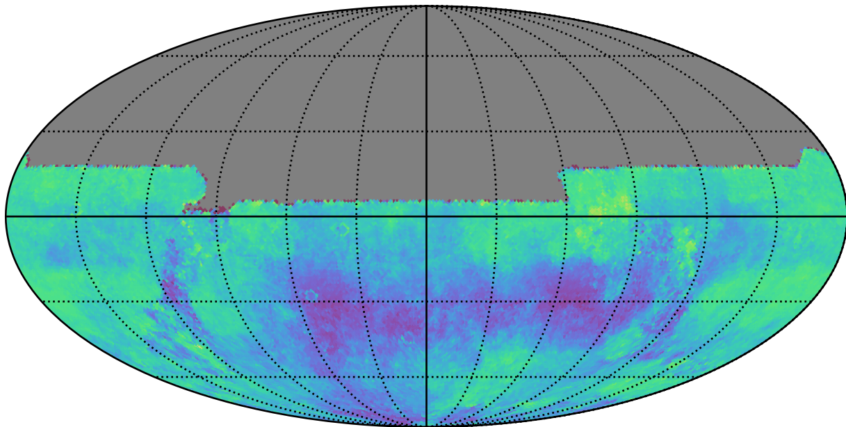
weather_cloudso30v3.4_10yrs u: Kuiper rotSkyPos
