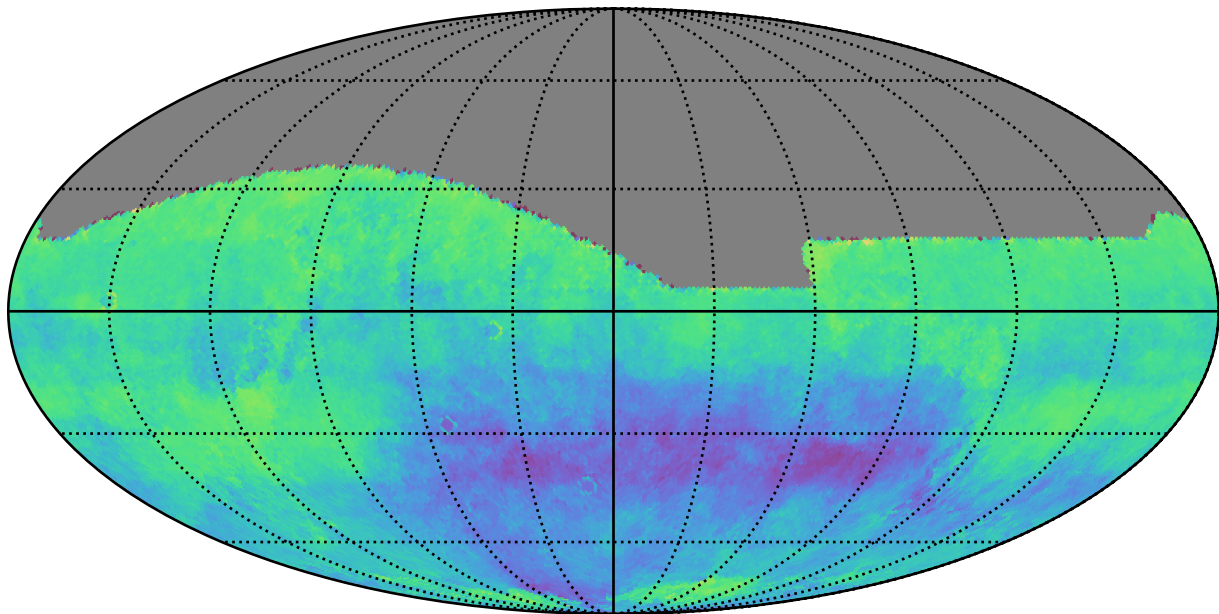
weather_cloudso30v3.4_10yrs i: Kuiper rotSkyPos
