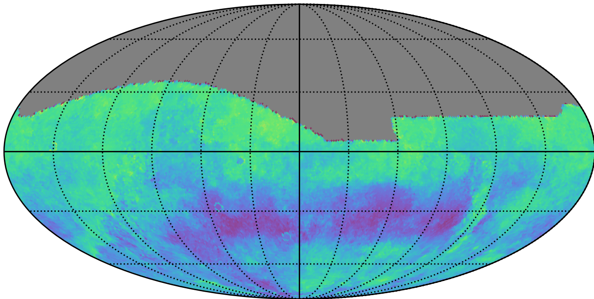
weather_cloudso30v3.4_10yrs g: Kuiper rotSkyPos
