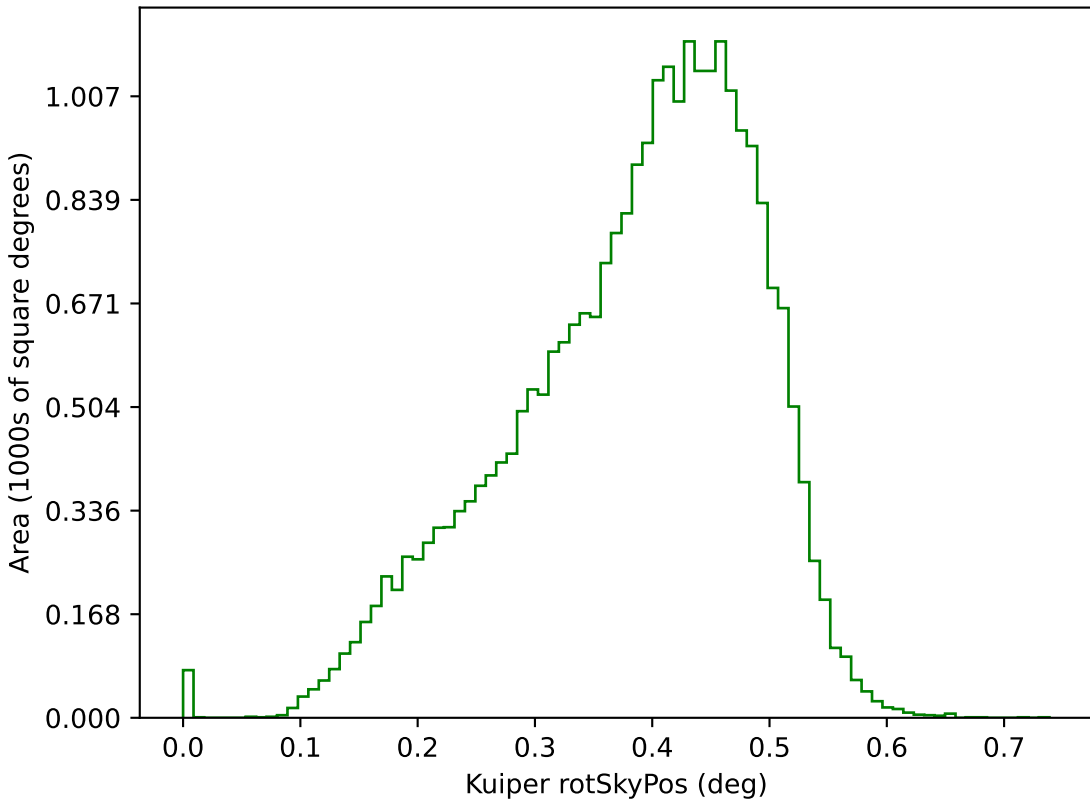
weather_cloudso30v3.4_10yrs g: Kuiper rotSkyPos
