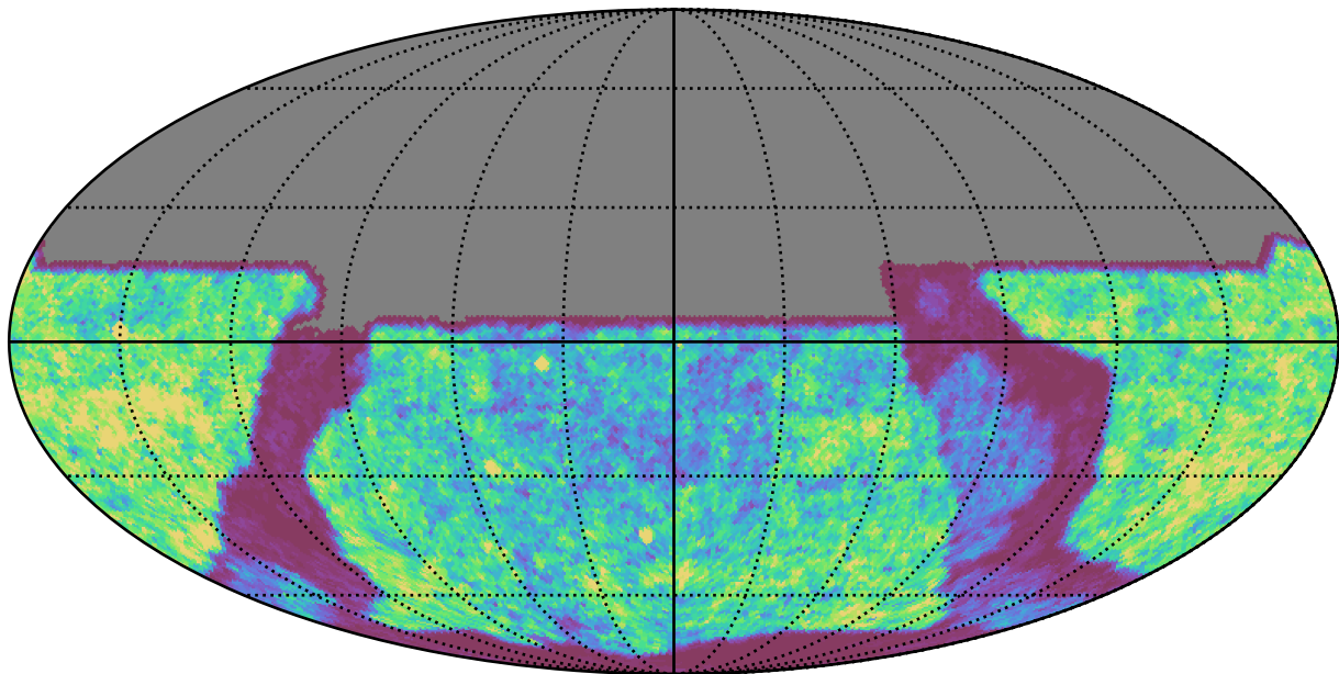
weather_cloudso30v3.4_10yrs y band: Gaps_24hr
