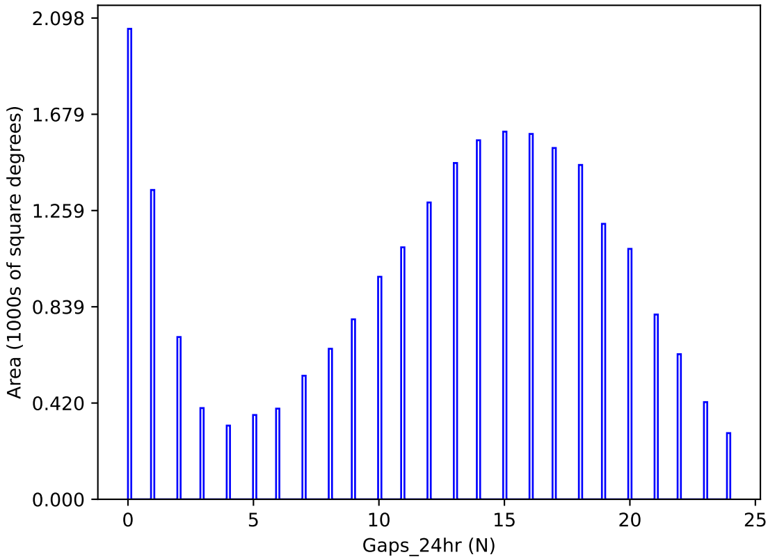
weather_cloudso30v3.4_10yrs y band: Gaps_24hr
