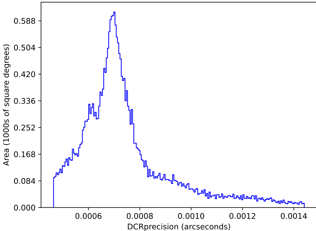
weather_cloudso30v3.4_10yrs : DCRprecision
