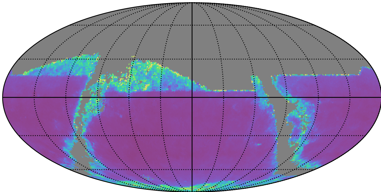
weather_cloudso30v3.4_10yrs z band: AGN SF_uncert
