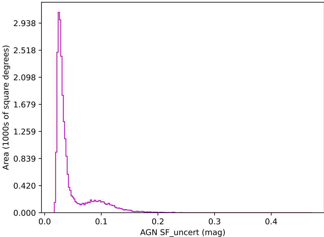
weather_cloudso30v3.4_10yrs z band: AGN SF_uncert
