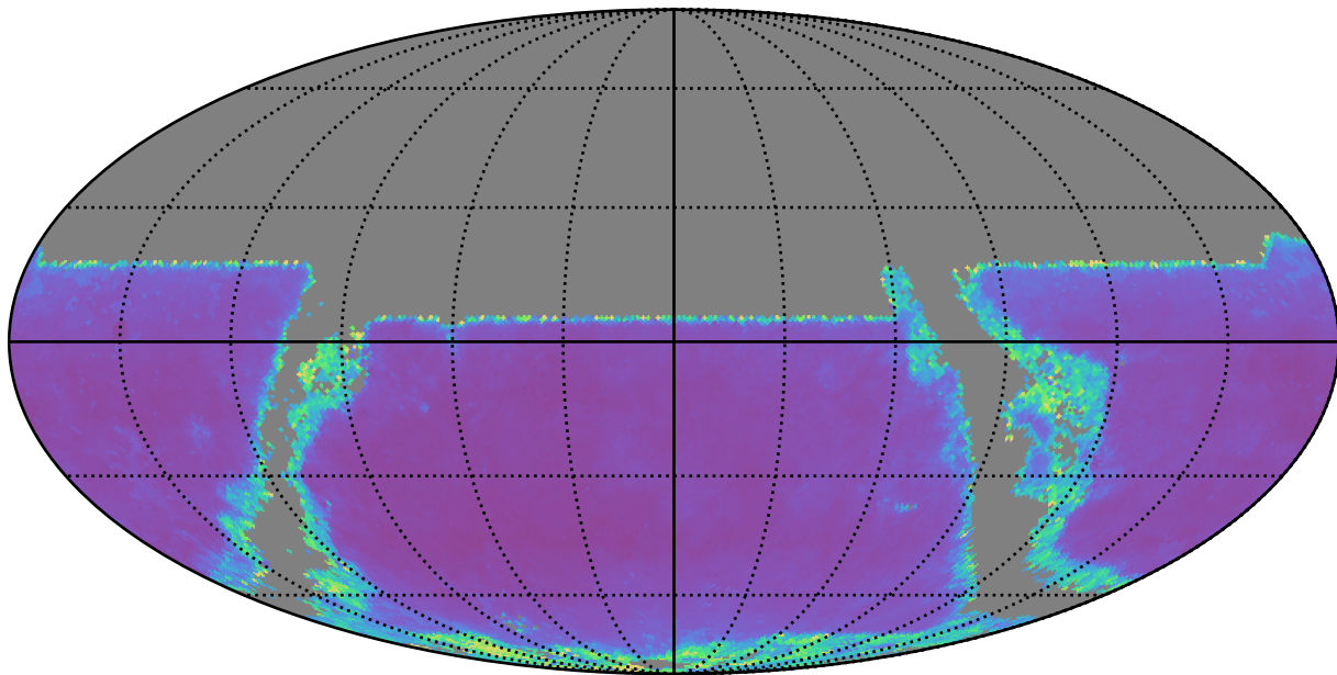
weather_cloudso30v3.4_10yrs y band: AGN SF_uncert
