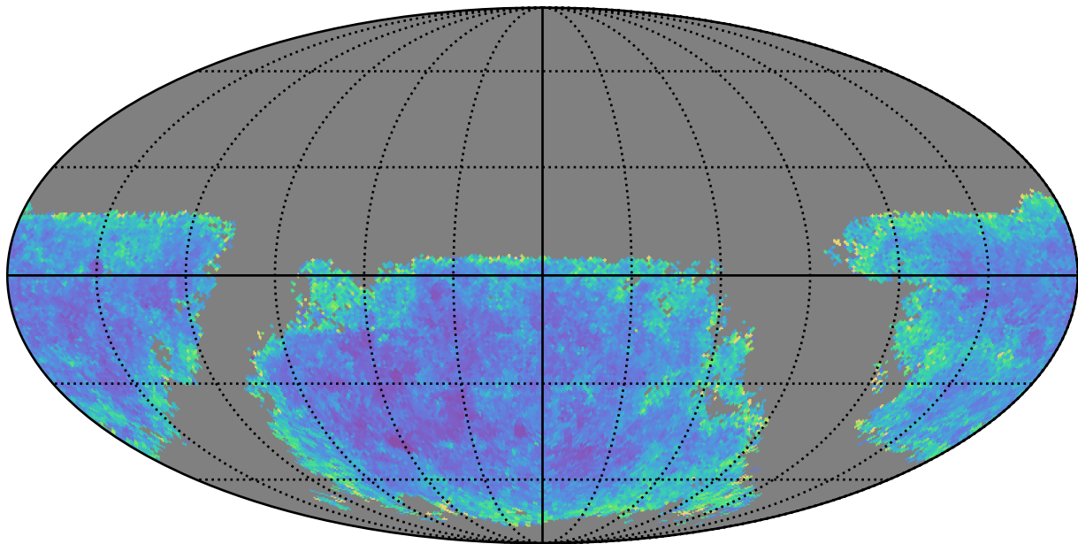
weather_cloudso30v3.4_10yrs u band: AGN SF_uncert
