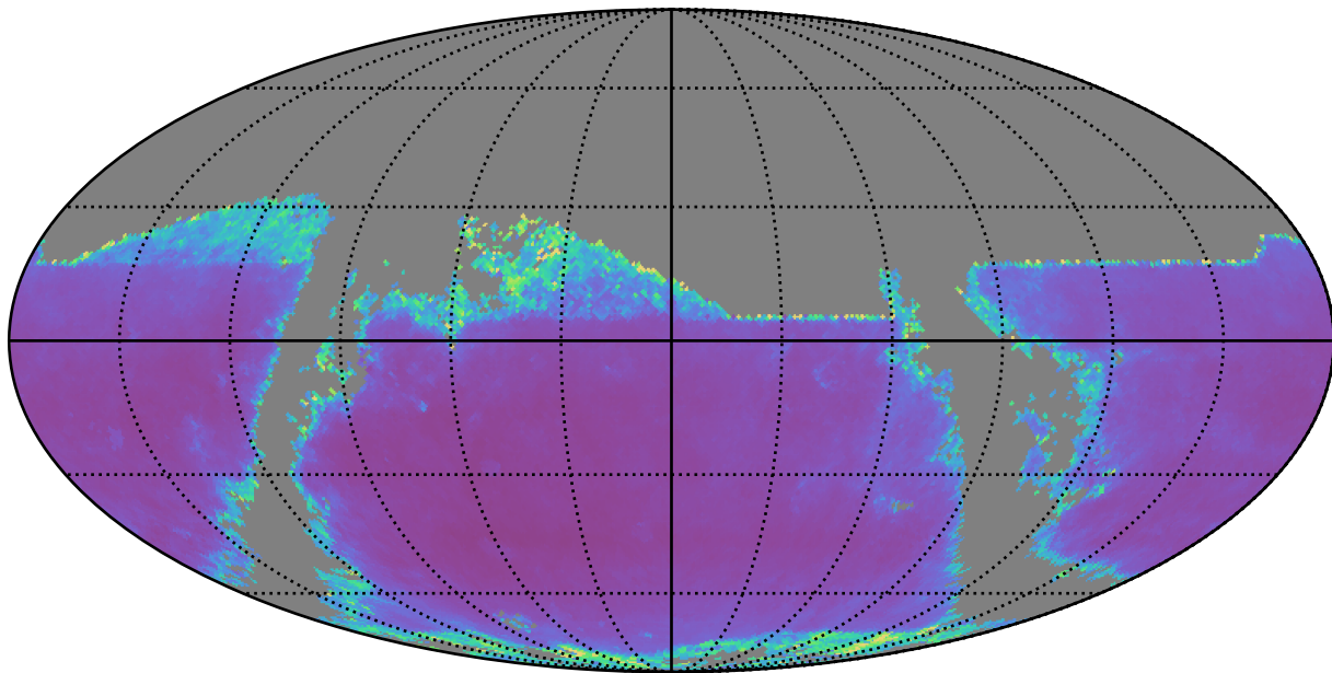
weather_cloudso30v3.4_10yrs r band: AGN SF_uncert
