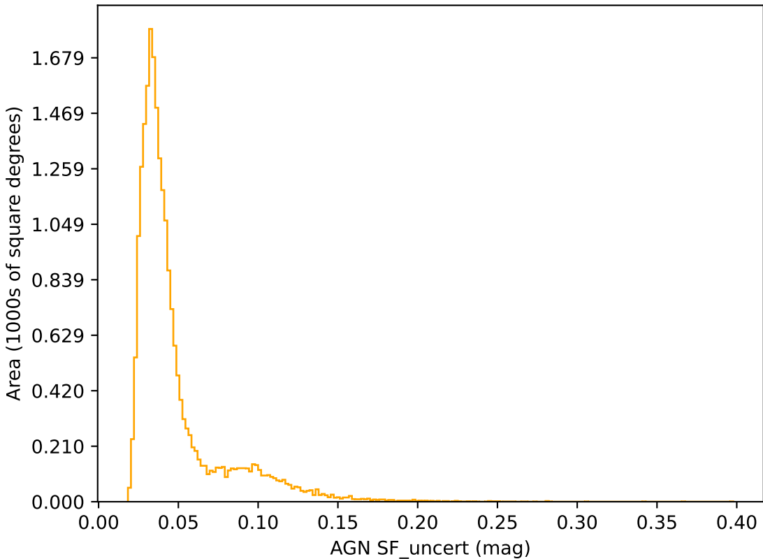
weather_cloudso30v3.4_10yrs r band: AGN SF_uncert
