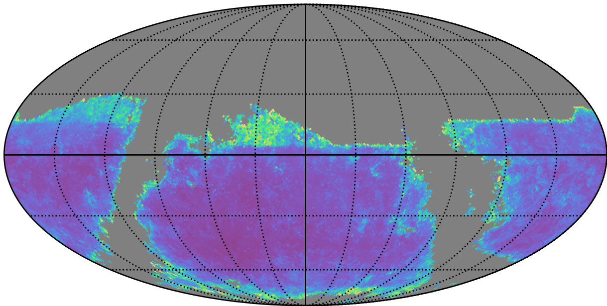
weather_cloudso30v3.4_10yrs g band: AGN SF_uncert
