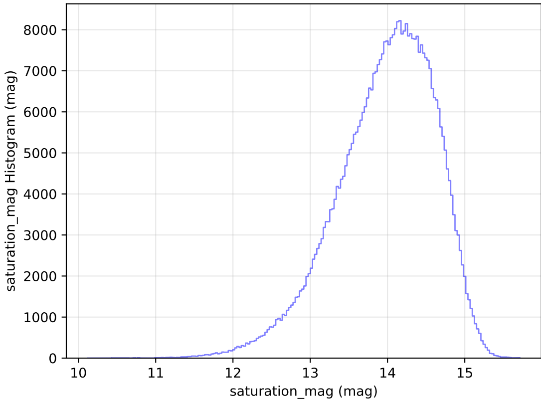
weather_cloudso30v3.4_10yrs WFD z band: saturation_mag Histogram
