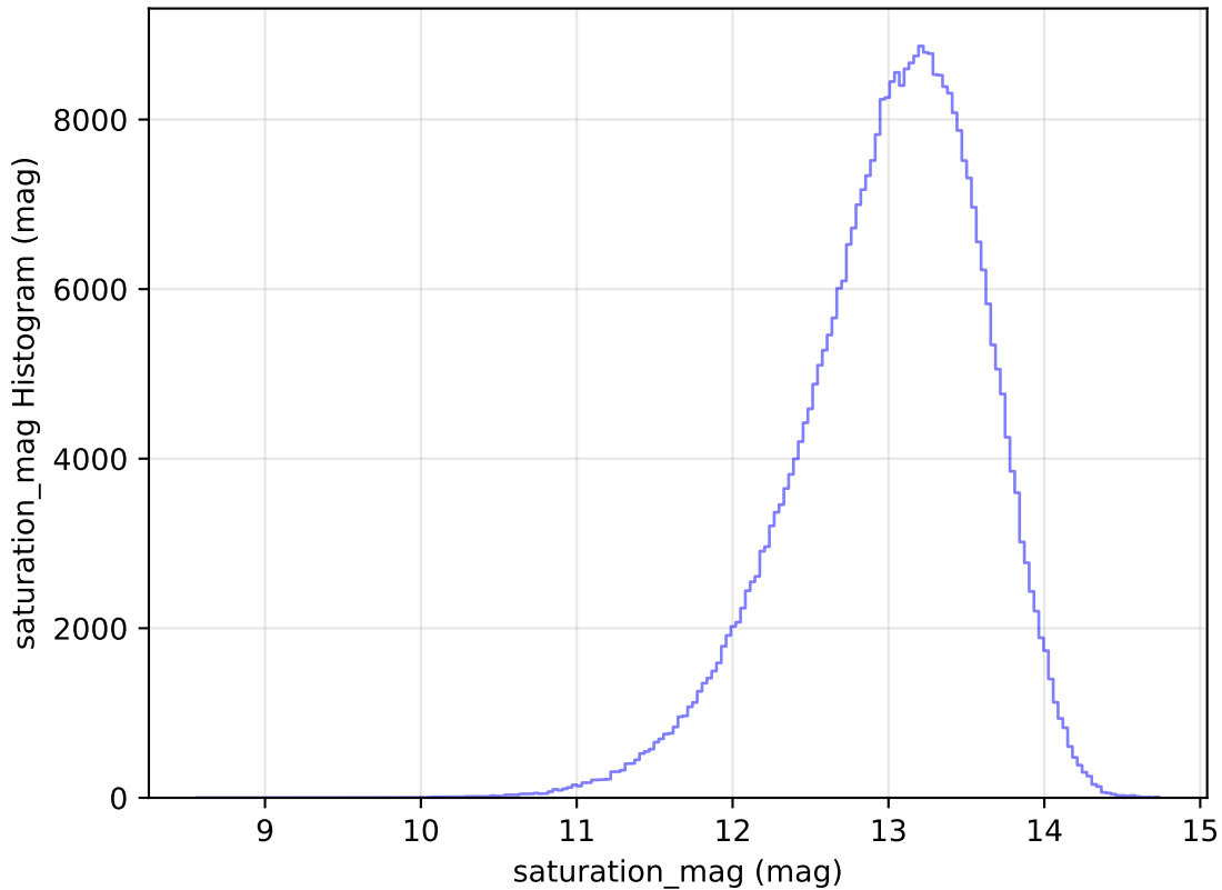
weather_cloudso30v3.4_10yrs WFD y band: saturation_mag Histogram
