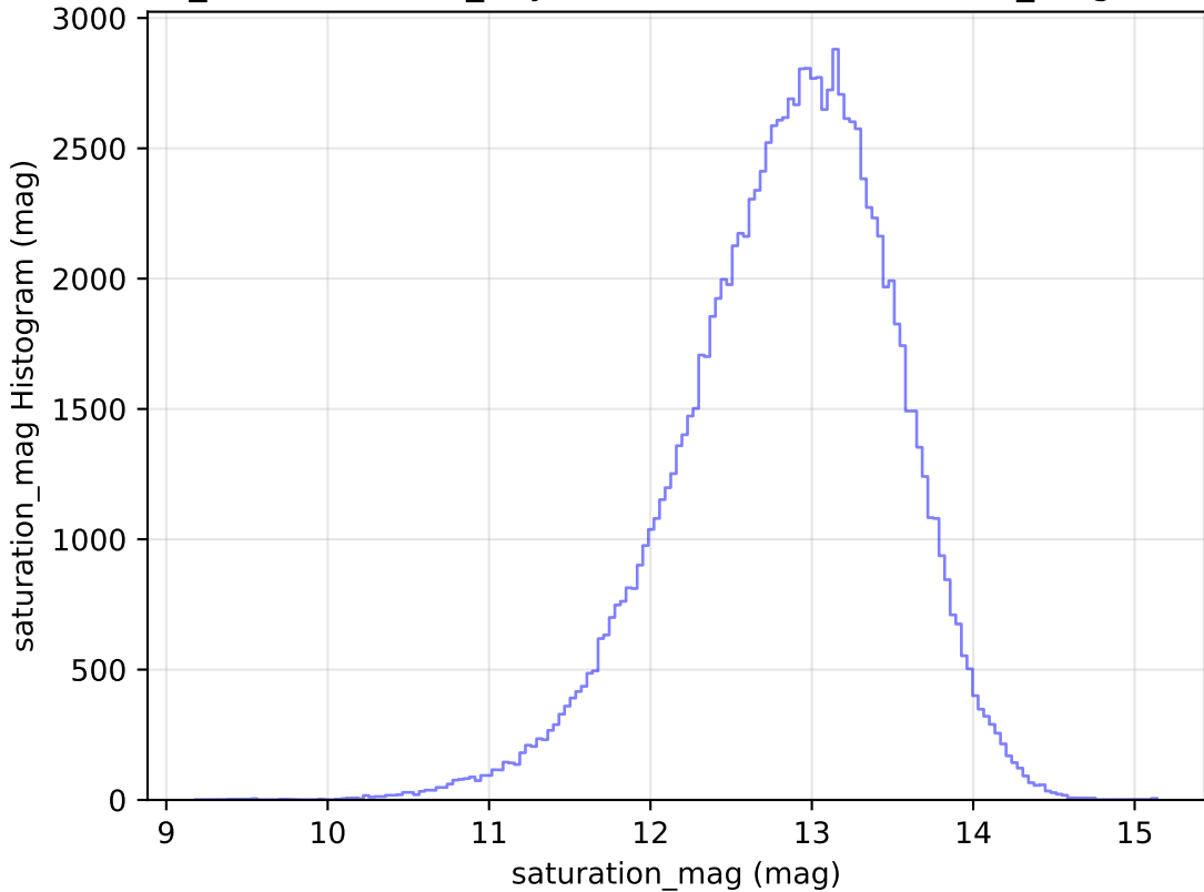
weather_cloudso30v3.4_10yrs WFD u band: saturation_mag Histogram
