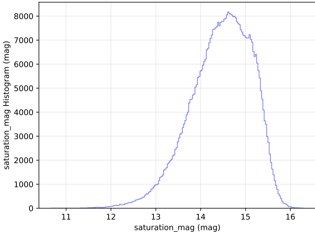
weather_cloudso30v3.4_10yrs WFD r band: saturation_mag Histogram
