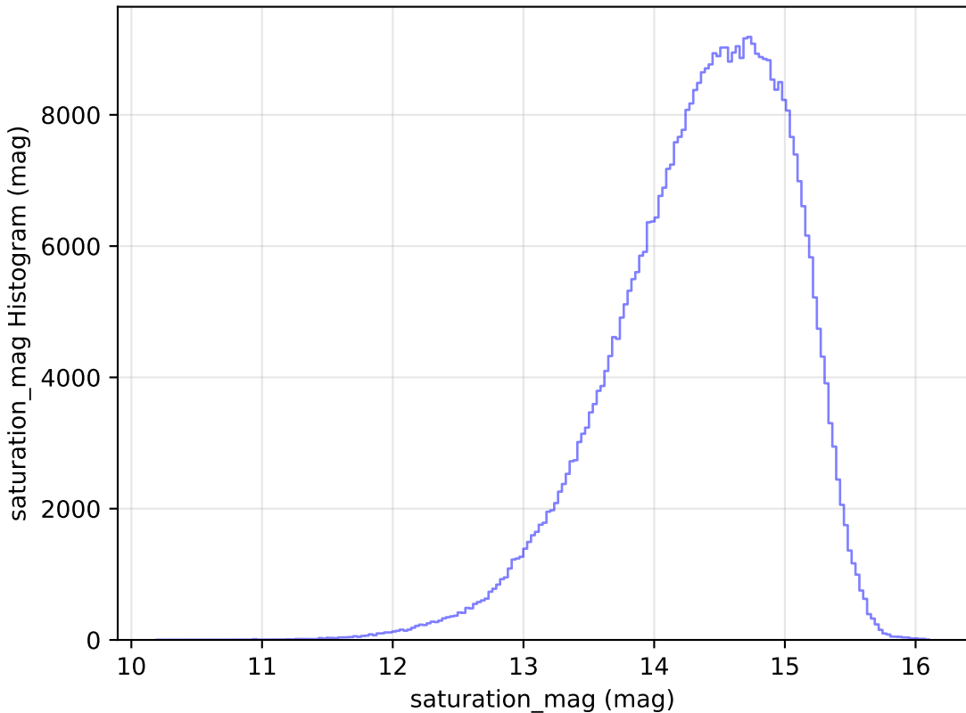
weather_cloudso30v3.4_10yrs WFD i band: saturation_mag Histogram
