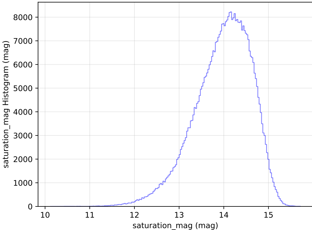
weather_cloudso30v3.4_10yrs All sky z band: saturation_mag Histogram
