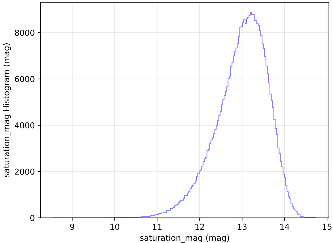
weather_cloudso30v3.4_10yrs All sky y band: saturation_mag Histogram
