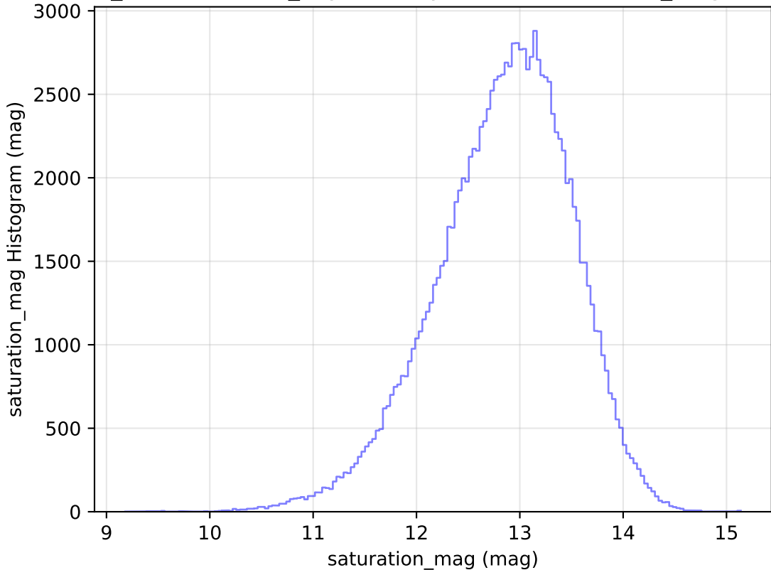
weather_cloudso30v3.4_10yrs All sky u band: saturation_mag Histogram
