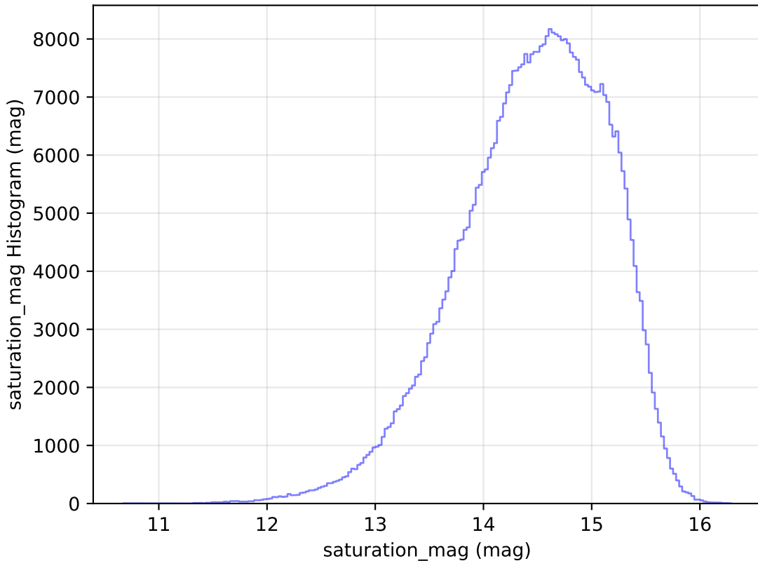
weather_cloudso30v3.4_10yrs All sky r band: saturation_mag Histogram
