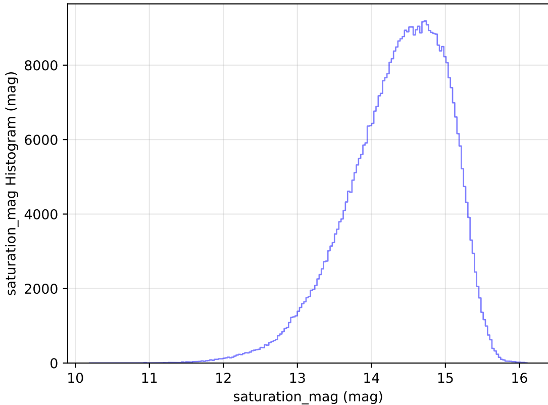
weather_cloudso30v3.4_10yrs All sky i band: saturation_mag Histogram
