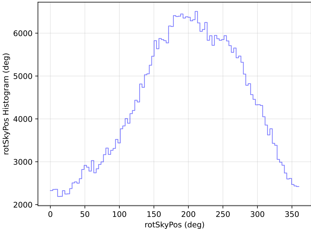
weather_cloudso30v3.4_10yrs WFD z band: rotSkyPos Histogram
