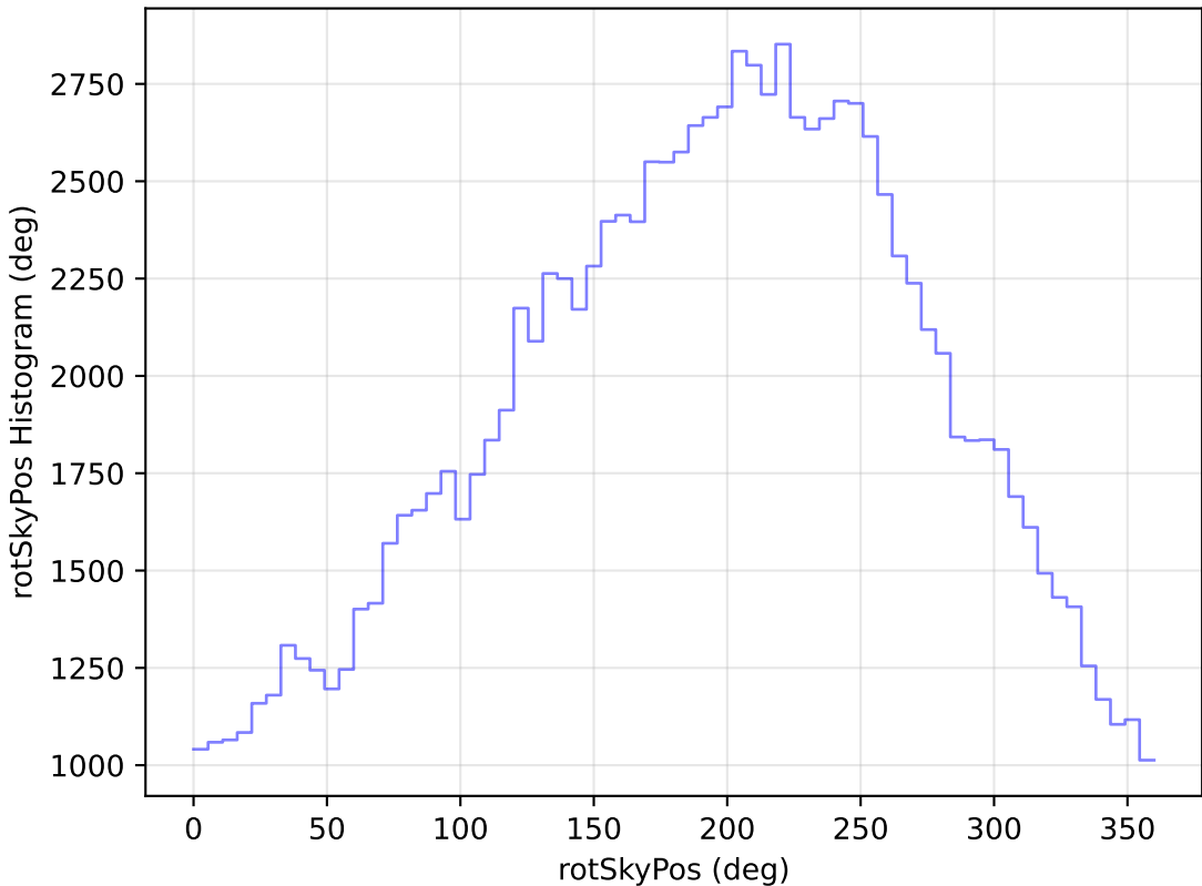
weather_cloudso30v3.4_10yrs WFD u band: rotSkyPos Histogram
